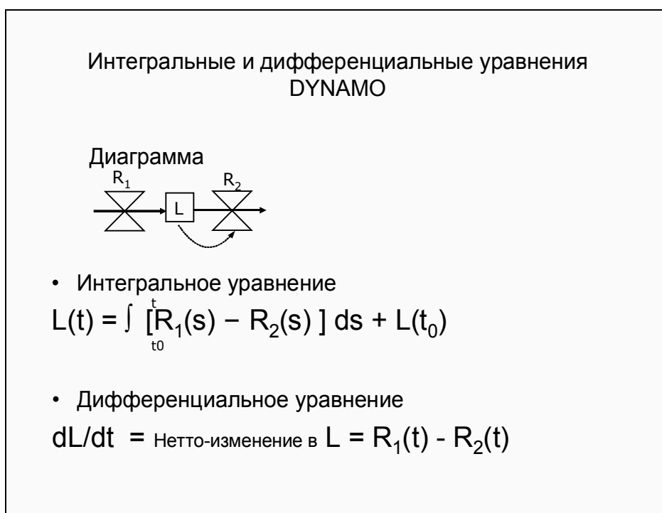
Рис.2.2. Уравнения компилятора DYNAMO
